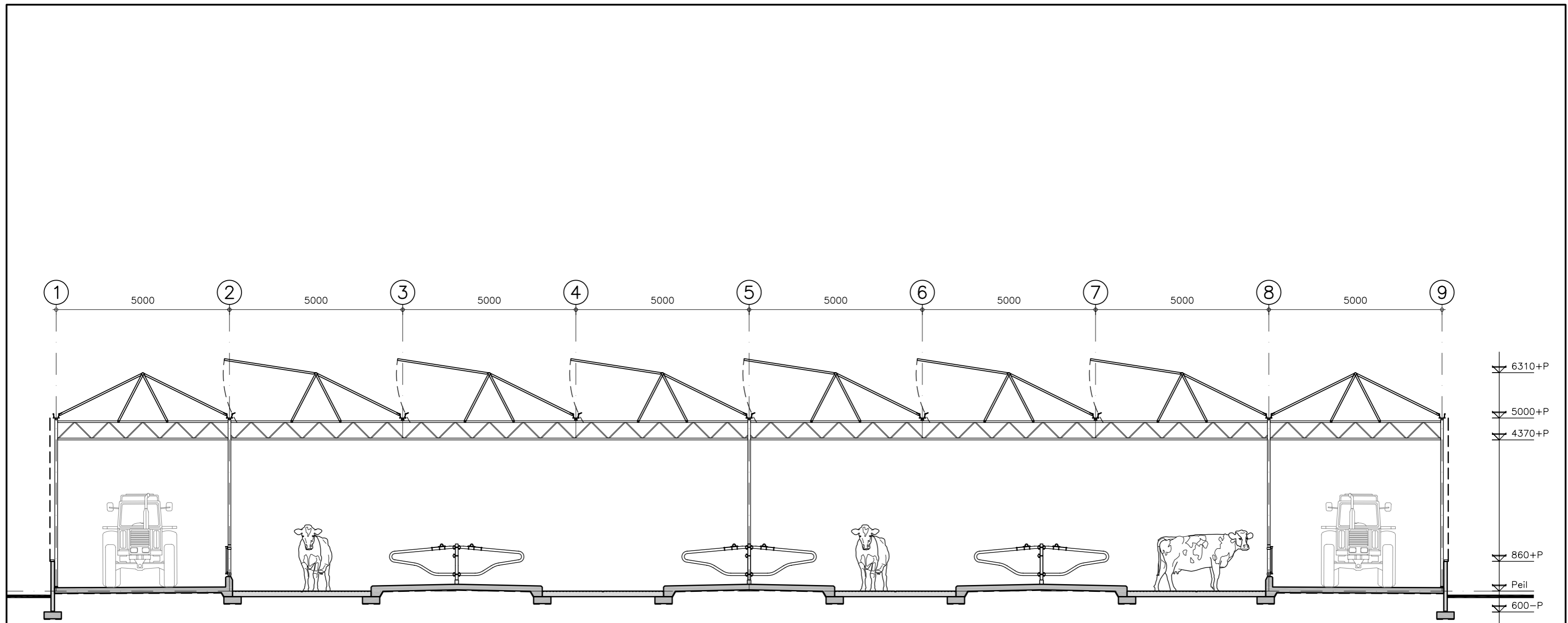
Doorsnede
